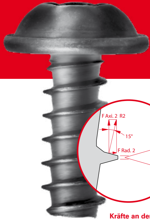
Kräfte an der Gewindeflanke
