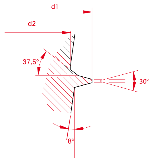
Gewindegang vergrößert
